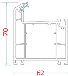
GNC - 621 - F02 Door Outer Frame
