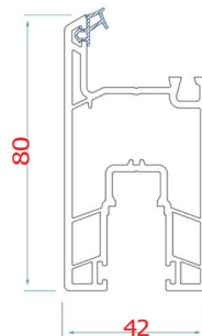
GNS - 621 - S03 Door Sash
