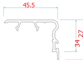
GNS - 620 - L02 Interlock for Door Sash
