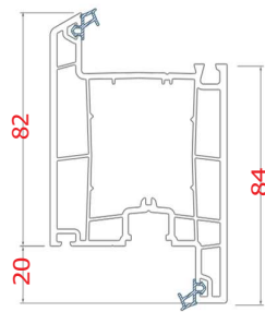
GNC - 621 - S04 Inward Opening Door Sash
